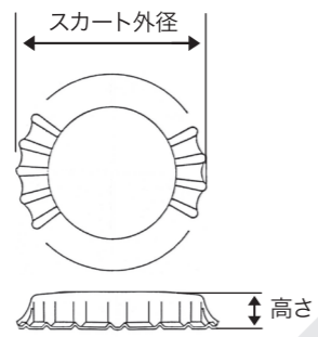
キャップ 寸法参考
