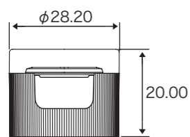
キャップ寸法
