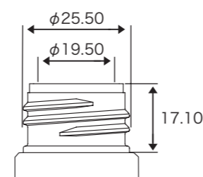
対象容器口寸法
