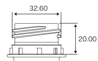
対象容器口寸法
